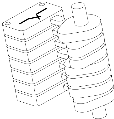
Abbildung 10: Nockenendschalter
