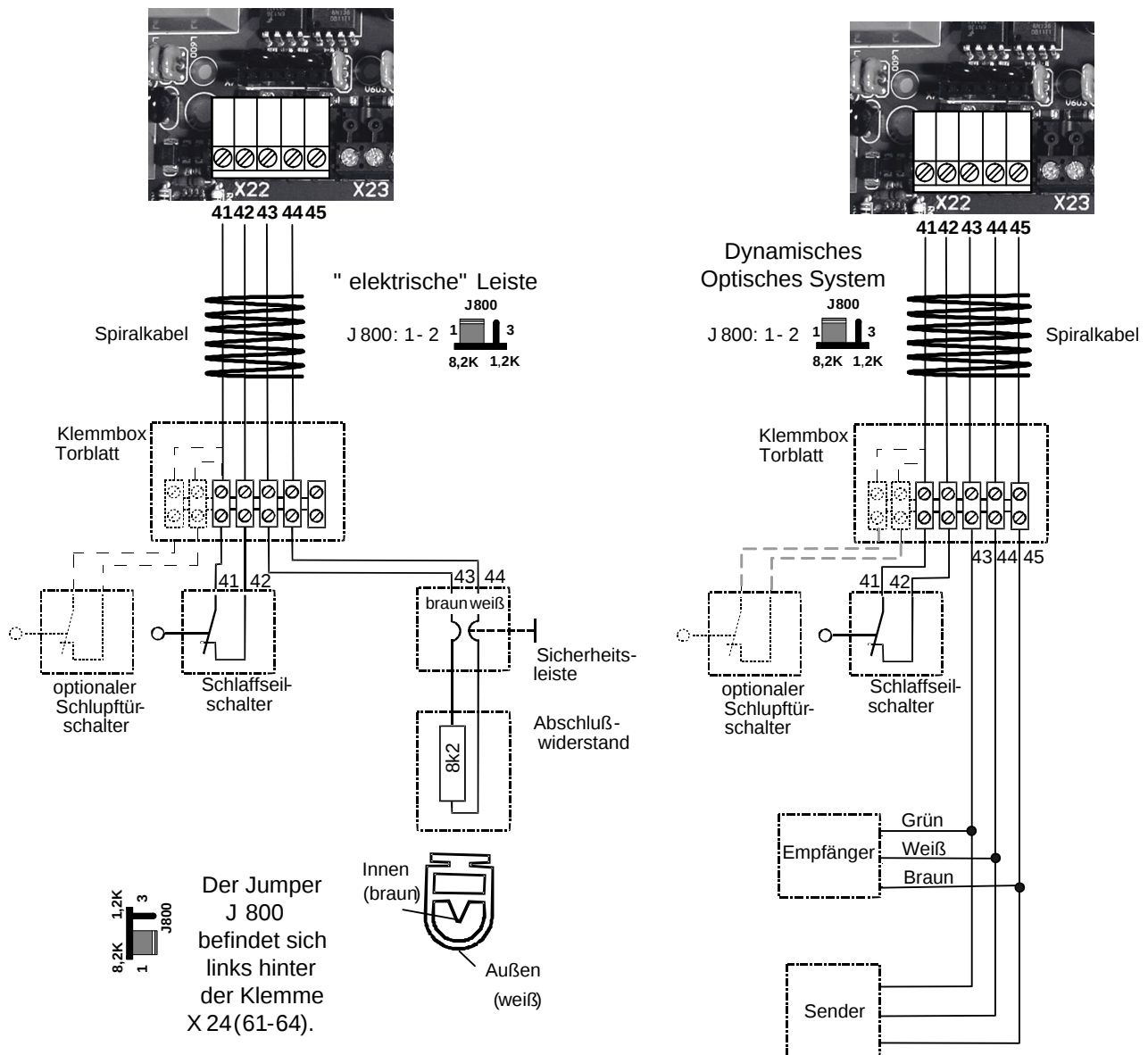
Abbildung 6: Anschluss der Sicherheitsleiste
