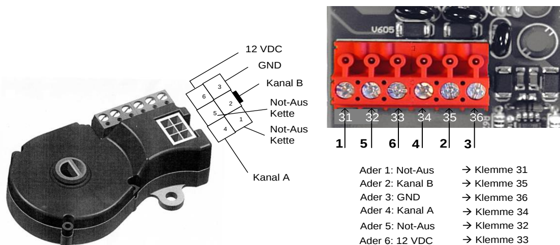
Abbildung 9: Anschluss Absolutwertgeber DES
