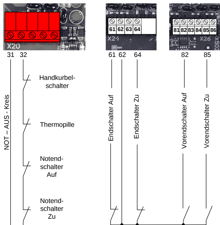
Abbildung 11: Anschluss Nockenendschalter
