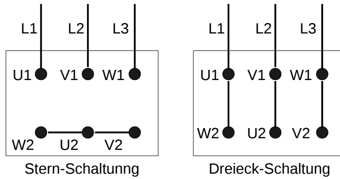
Abbildung 19: Stern- / Dreieckschaltung
